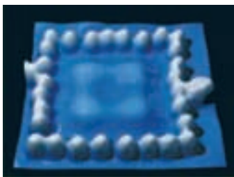
Μια νησίδα πυριτίου πάνω σε κρύσταλλο πυριτίου διαλύεται αργά στους 450 βαθμούς. Η γνώση των διεργασιών αυτών έχει σημασία για την ποιότητα των λεπτών στιβάδων.
