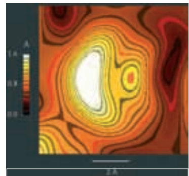
Στο μετωπιαίο άτομο ακίδας σάρωσης κρέμονται δύο νέφη ηλεκτρονίων, που διαγράφουν τροχιές ακριβώς όπως περιγράφεται στα διδακτικά βιβλία.
