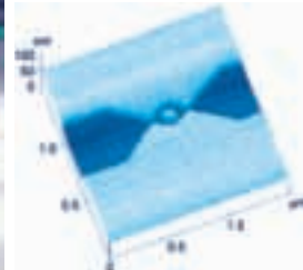
Εξάσκηση για τον κβαντικό υπολογιστή: ιντερφερόμετρο Aharanov-Bohm, που κατασκευάστηκε στο Πανεπιστήμιο του Ρουρ, Bochum, με μικροσκόπιο ατομικών δυνάμεων (AFM).
